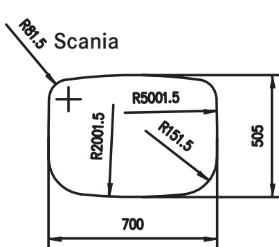
Material: Stahl/Steel Querschnitt/Cross section: F09
