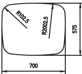
Material: Aluminium Querschnitt/Cross section: 991
