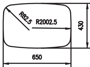
Material: Aluminium Querschnitt/Cross section: 881
