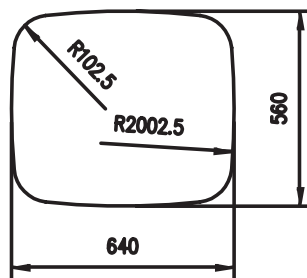
Material: Aluminium Querschnitt/Cross section: 931
