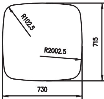
Material: Aluminium Querschnitt/Cross section: 501
