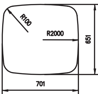
Material: Aluminium Querschnitt/Cross section:
