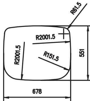
Material: Stahl/Steel Querschnitt/Cross section: F08
