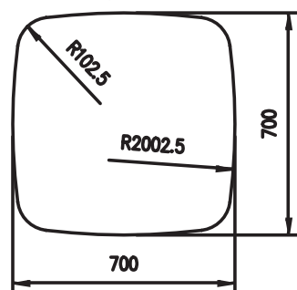
Material: Aluminium Querschnitt/Cross section: 963
