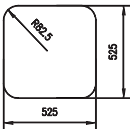
Material: Aluminium Querschnitt/Cross section: 821
