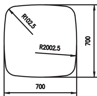
Material: Aluminium Querschnitt/Cross section: 953
